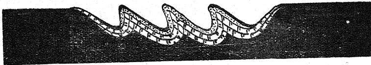
चित्र १६-चट्टानों का अधिक उमार
